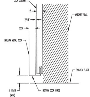
DETAIL D – BOTTOM DOOR GUIDE SECTION
